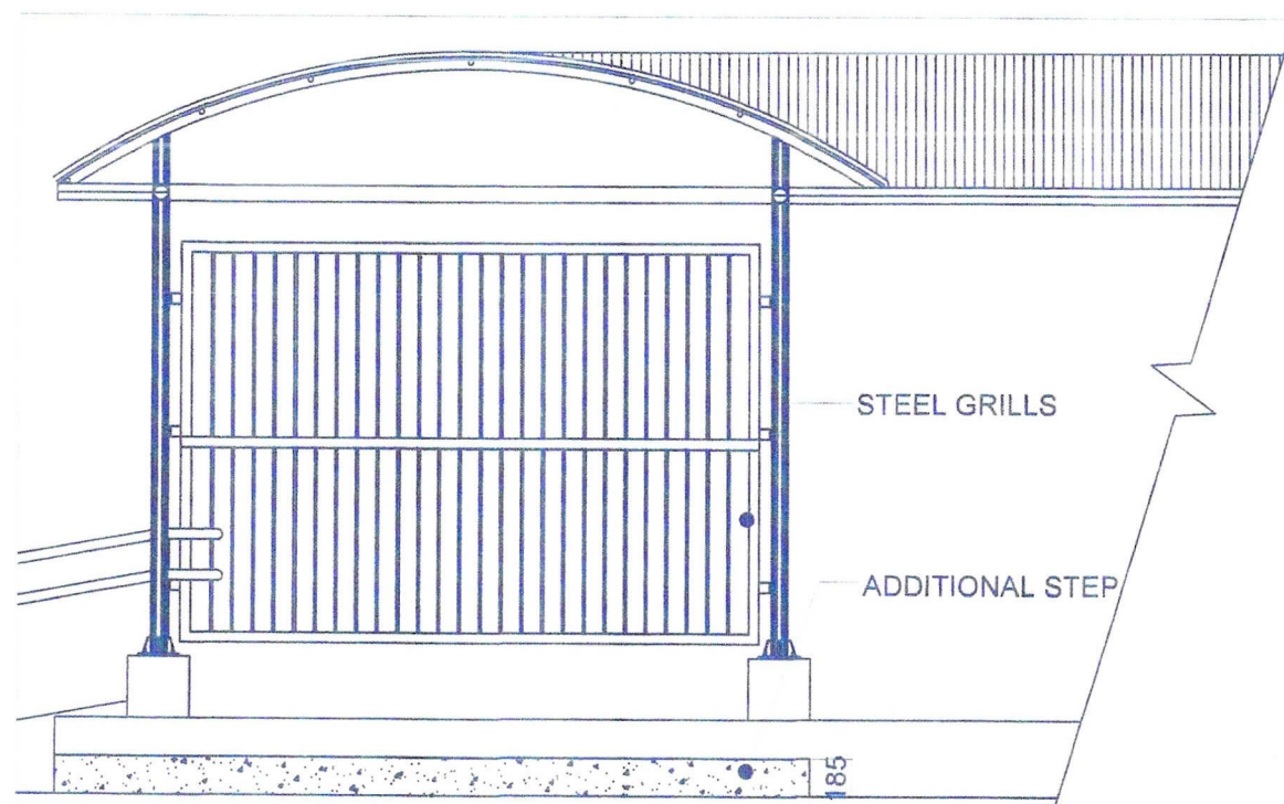
ELEVATION
